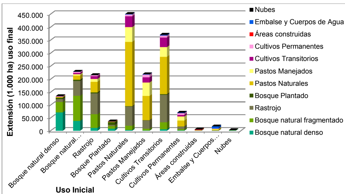
Gráfica 16. Extensión de los cambios para los usos en el subperíodo 1986-2000
