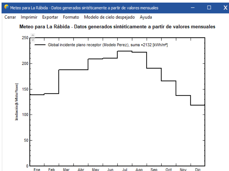
Figura 16. Plano inclinado global. Fuente: PVSyst.
