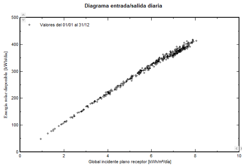
Figura 23. Diagrama entrada/salida diaria, Zona I. Fuente: PVSyst.
